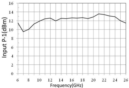
Input P-1@LO=13dBm
