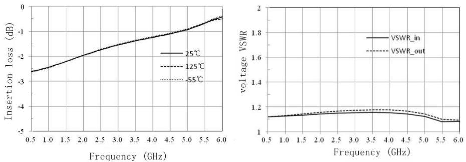
CW-AE00506-2 (bondwire)
