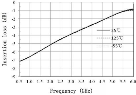
CW-AE00506-6 (bondwire)
