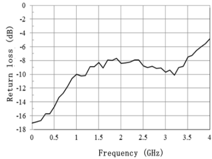
IF return loss
